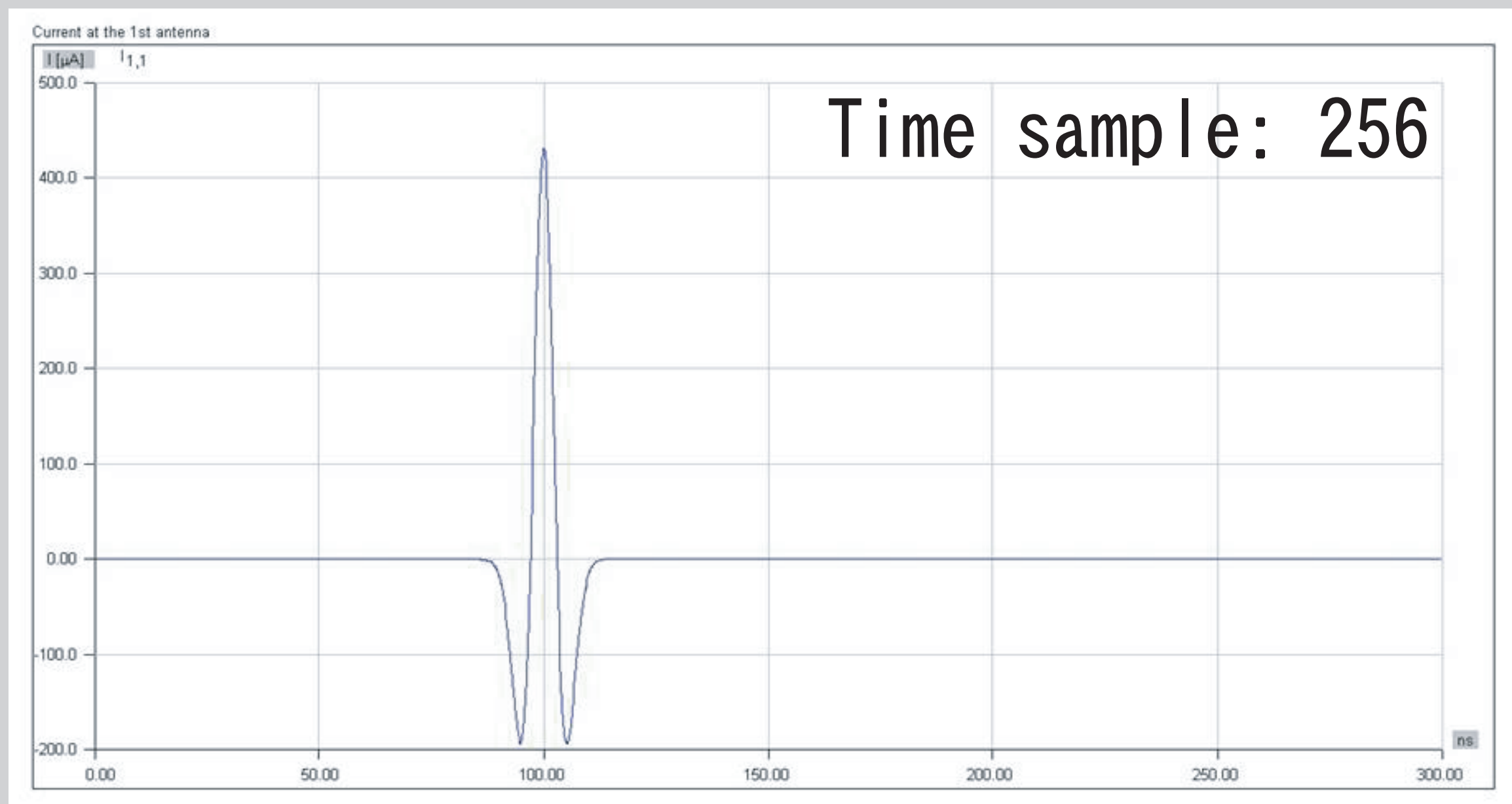
励振パルスの電流波形
